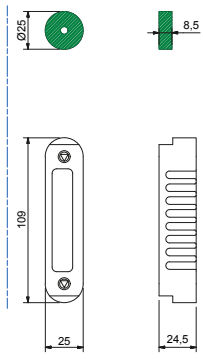
Opvulling t.b.v. Verstelbare Sluitplaat Art. nr. 700006 Spacer ring for Adjustable Strike Sluitkom Nachtschoot Art. nr. 707022 (Din Ls/Rs) Casing for Adjustable Strike Deadbolt
