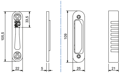
Verstelbare Sluitplaat Haakschoot Art. nr. 600357 Adjustable Strike for Hookbolt
