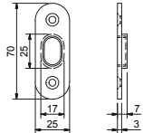
Magneet voor MPS (Auto)Motortronic Art. nr. 200076 Magneet for MPL's (Auto)Motortronic
