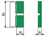
Verlengblokjes voor Verst. Sluitpl. Art. nr. 600599 (16 mm) Art. nr. 600598 (12 mm) Art. nr. 600597 (8 mm) Art. nr. 600596 (4 mm) Strike Extenders (size)
