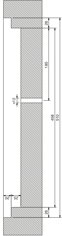
A-A (1:2)
