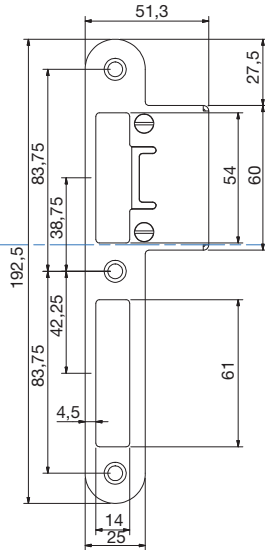
Nastelbare sluitplaat, magneet en sluitkom t.b.v. Automatic dagschoot Art. 706440(1) + 200089(2) + 707021(3)
