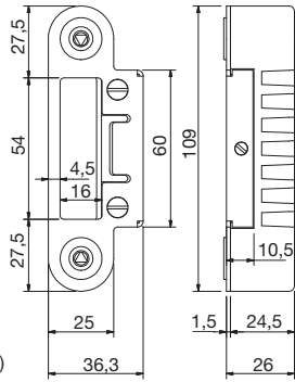
Nastelbare sluitplaat, magneet en sluitkom t.b.v. Automatic dagschoot Art. 706440(1) + 200089(2) + 707021(3)
