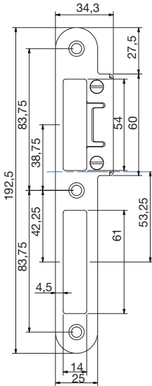
Nastelbare sluitplaat, magneet en sluitkom t.b.v. Automatic dagschoot Art. 706440(1) + 200089(2) + 707021(3)
