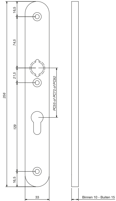
Afb. 3 Smal beslag
