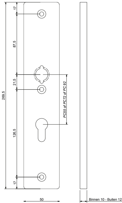
Afb. 2 Breed beslag
